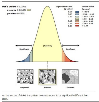
شکل ۱۱. منحنی همبستگی فضایی موران و Z-score و P-value برای کاربری ورزشی
