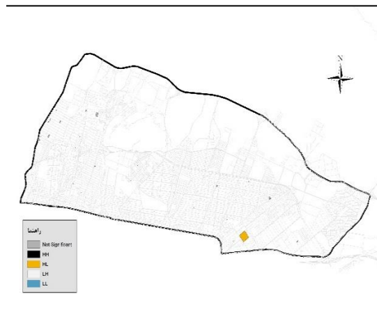
شکل ۸. خروجی مدل فضایی موران برای کاربری فرهنگی در سطح منطقه ۴
