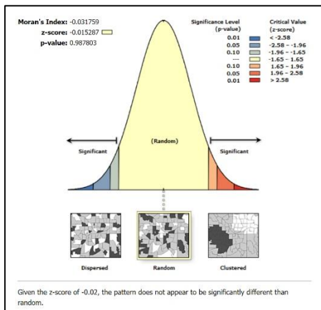
شکل ۹. منحنی همبستگی فضایی موران و Z-score و P-value برای کاربری فرهنگی
