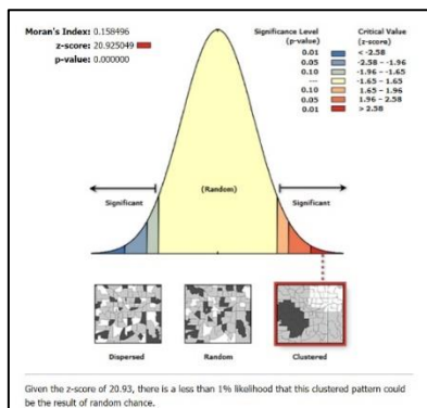
شکل ۵. منحنی همبستگی فضایی موران و Z-score و P-value برای کاربری فضای سبز و پارک‌ها
