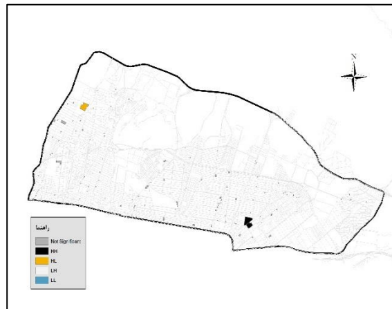
شکل ۱۴. خروجی مدل فضایی موران برای کاربری بهداشتی-درمانی در سطح منطقه ۴
