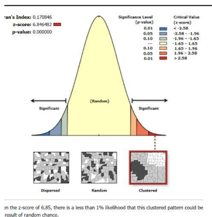
شکل ۱۵. منحنی همبستگی فضایی موران و Z-score و P-value برای کاربری آموزشی
