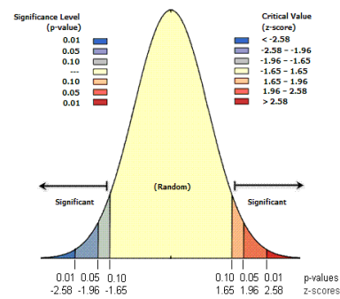
شکل ۱. مقادیر استاندارد Z-score و P-value
