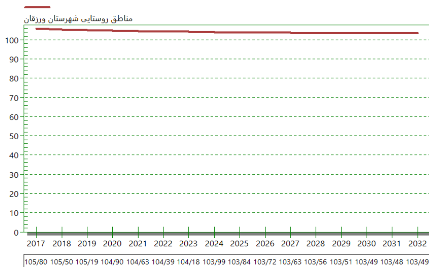
شکل ۳- نمودار آینده‌نگری نسبت جنسی جمعیت در مناطق روستایی شهرستان ورزقان
