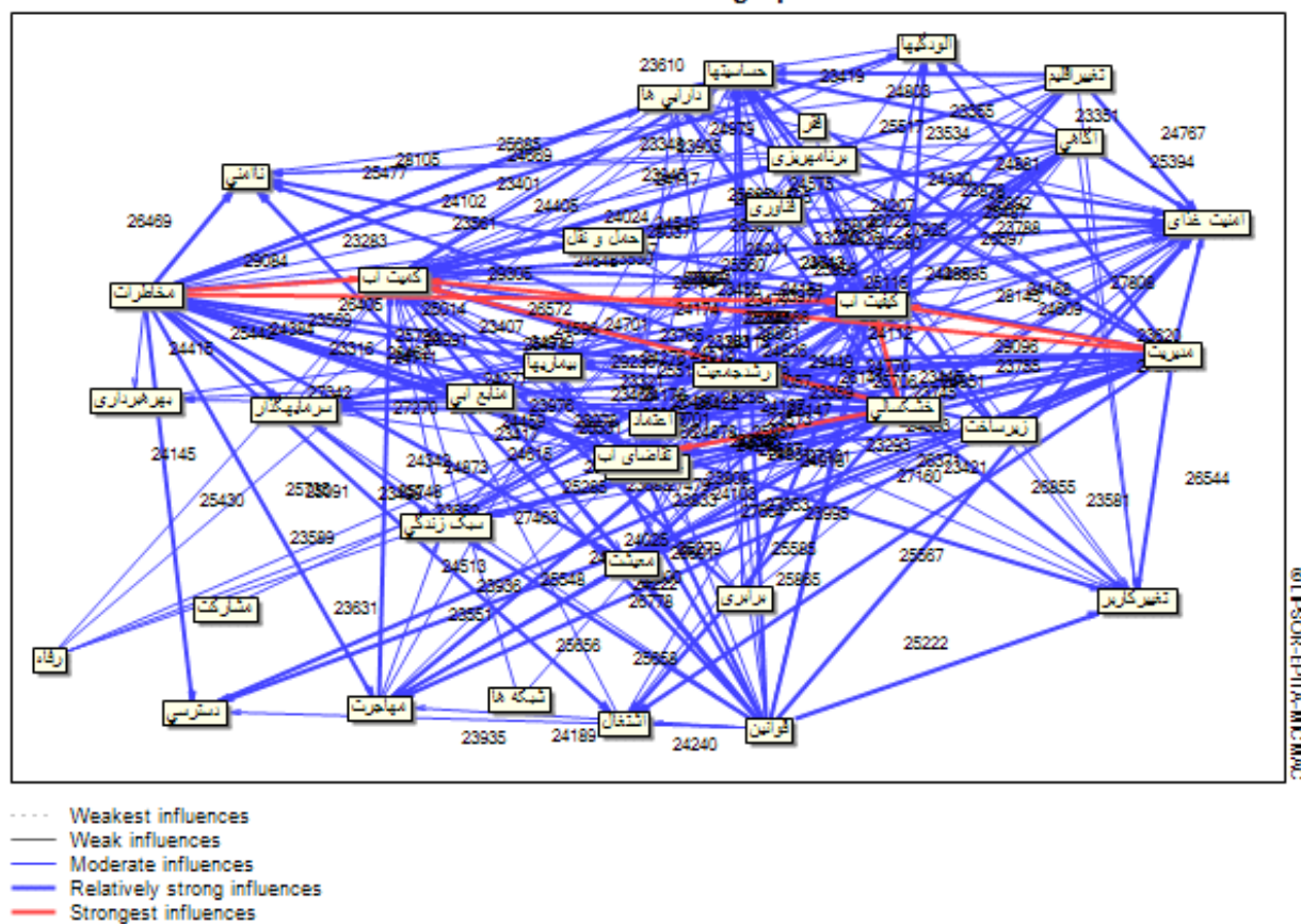
شکل ۸. گراف روابط غیرمستقیم بین متغیرها (منبع: نگارنده، ۱۴۰۲).
