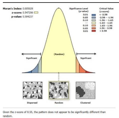
شکل ۷. منحنی همبستگی فضایی موران و Z-score و P-value برای کاربری مذهبی
