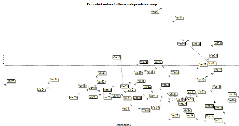
شکل ۵. رابطه مستقیم بین متغیرهای تأثیرگذار، دوجویی، تأثیرپذیر، مستقل و تنظیمی (پراکندگی متغیرها و جایگاه آن ها در محور تأثیرگذاری- تأثیرپذیری) (خروجی نرم افزار MICMAC) (مأخذ: یافته های پژوهش، ۱۴۰۴)
