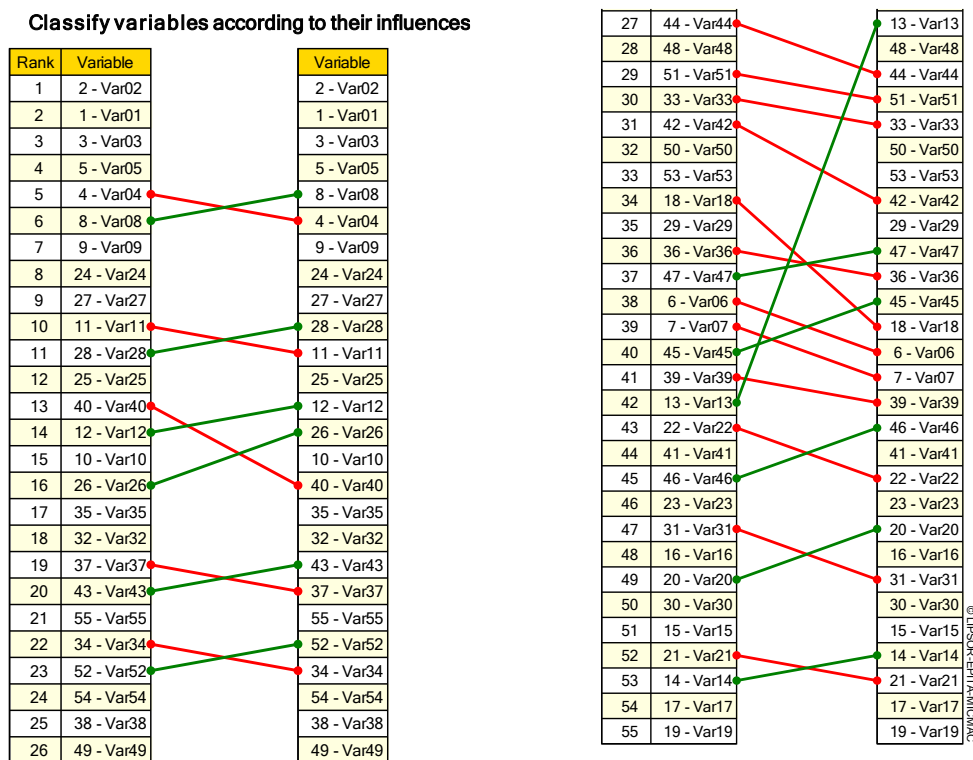
شکل ۸. نمودار جابه جایی شاخص های به دست آمده از الگوهای بالقوه مستقیم و غیرمستقیم (خروجی نرم افزار MICMAC) (مأخذ: یافته های پژوهش، ۱۴۰۴)
