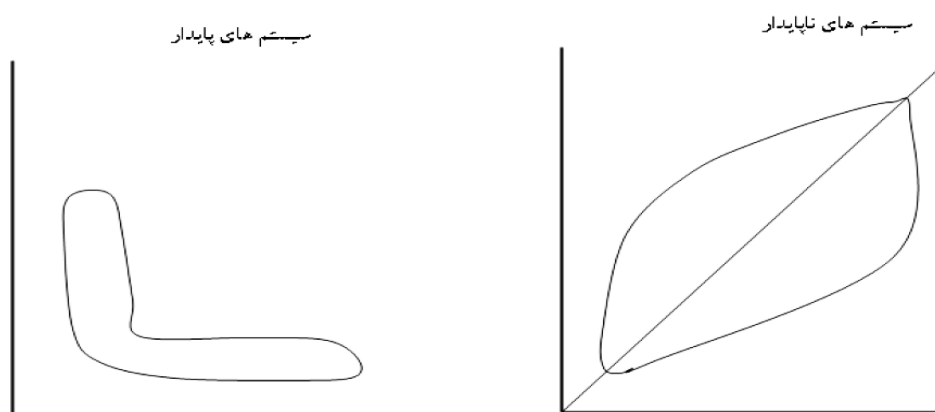
شکل ۳. نمودار پایداری یا ناپایداری سیستم (گودت و همکاران، ۲۰۱۱)
