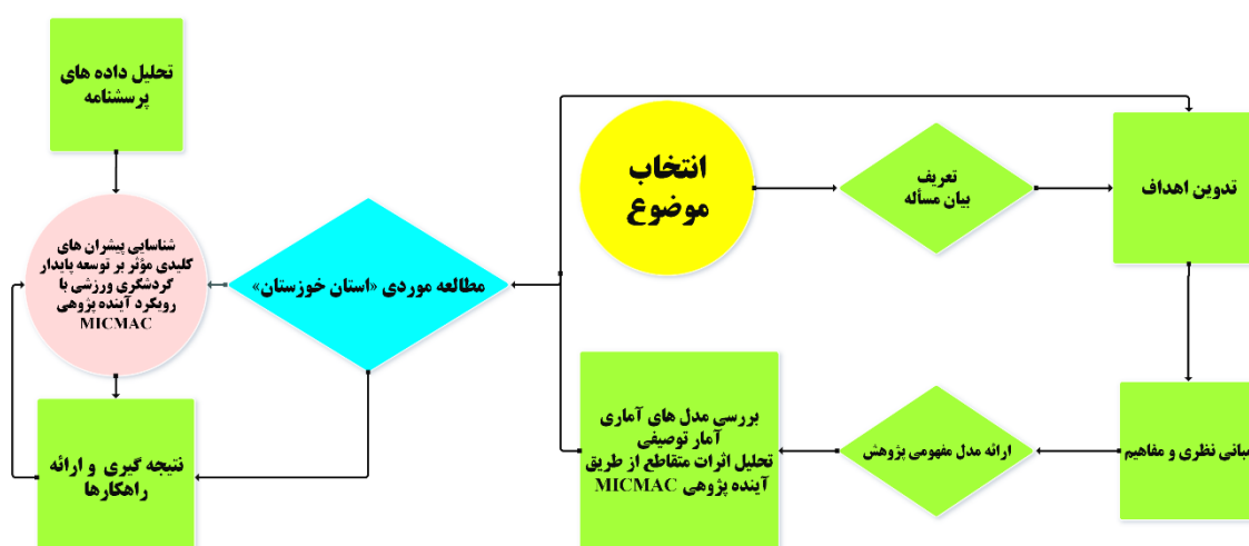
شکل ۴. مدل مفهومی پژوهش (مأخذ: یافته های پژوهش، ۱۴۰۴)
