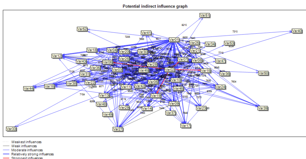
شکل ۷. نمودار پراکندگی متغیرها براساس تأثیرات غیرمستقیم بین متغیرها (خروجی نرم افزار MICMAC) (مأخذ: یافته های پژوهش، ۱۴۰۴)
