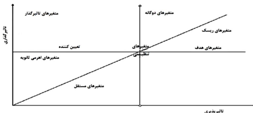
شکل ۲. تأثیرگذاری - تأثیرپذیری متغیرها در تحلیل اثرات متقاطع (گودت ۳ ، ۲۰۰۸)
