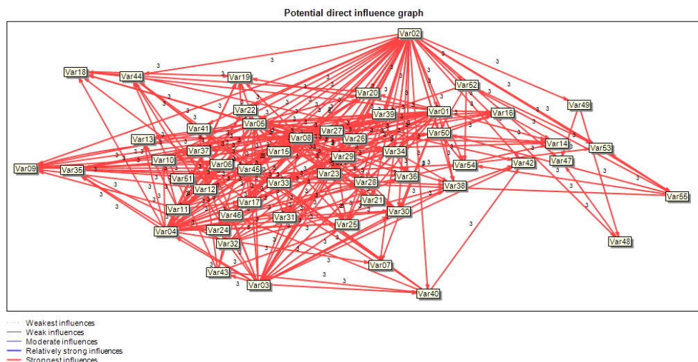
شکل ۶. نمودار پراکندگی متغیرها براساس تأثیرات مستقیم بین متغیرها (خروجی نرم افزار MICMAC) (مأخذ: یافته های پژوهش، ۱۴۰۴)
